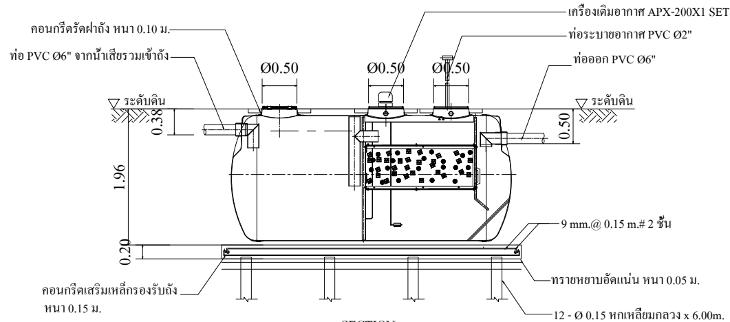
SECTION SCALE 1 : 100
