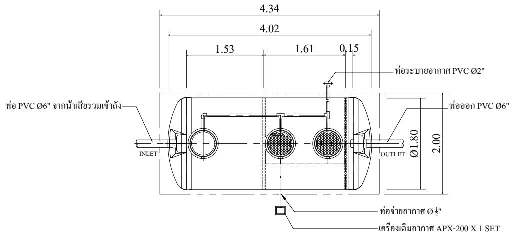
PLAN SCALE 1 : 100
