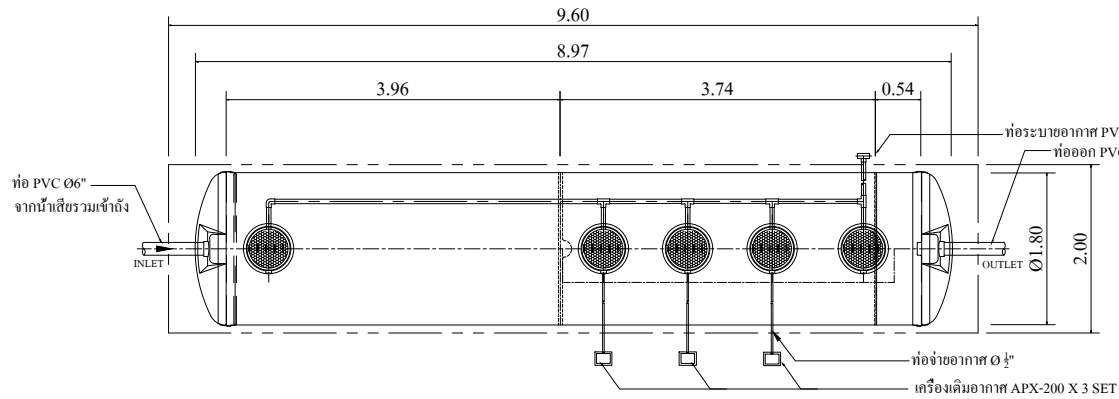
PLAN SCALE 1 : 100
