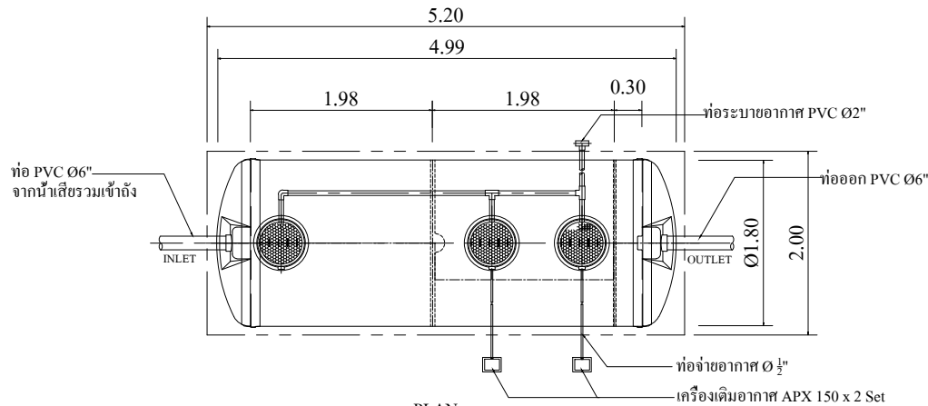
PLAN SCALE 1 : 100
