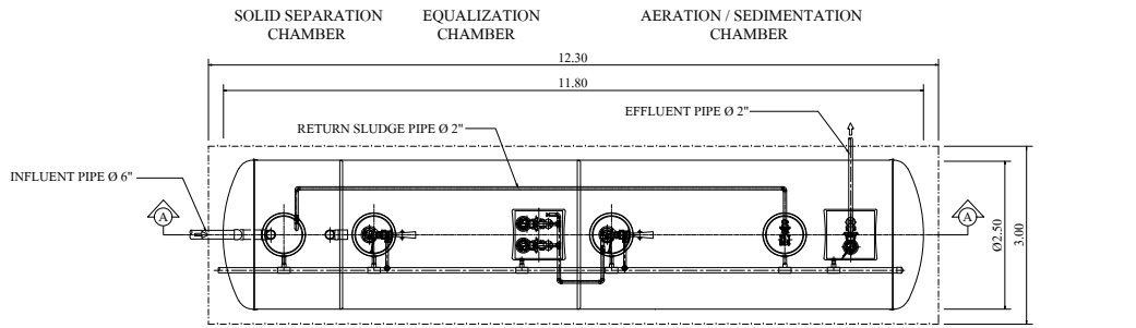
PLAN SCALE 1 : 100
