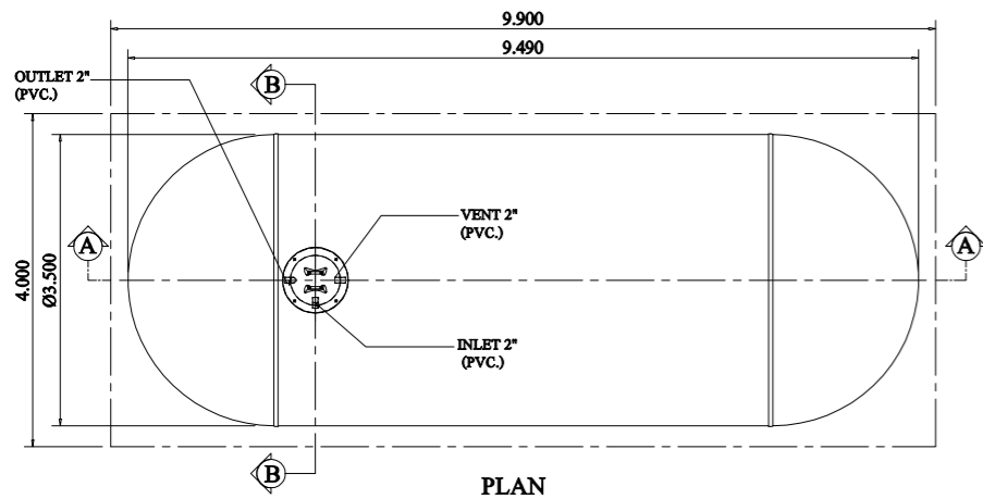
PLAN SCALE : 1:100
