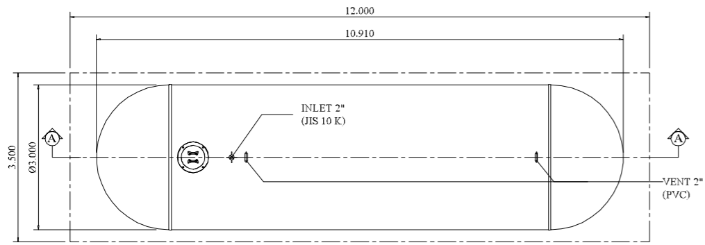
PLAN SCALE : 1:100
