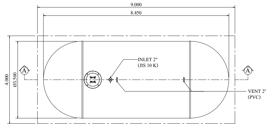
PLAN SCALE : 1:100
