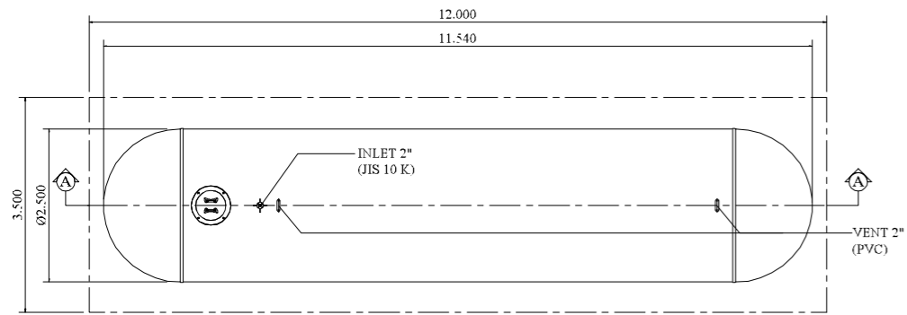
PLAN SCALE : 1:100
