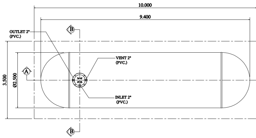
PLAN SCALE : 1:100
