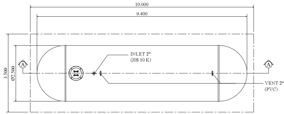
PLAN SCALE : 1:100
