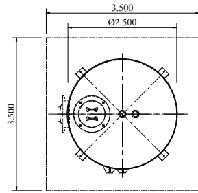
PLAN SCALE : 1:100
