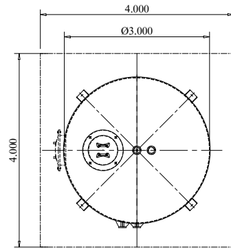
PLAN SCALE : 1:100
