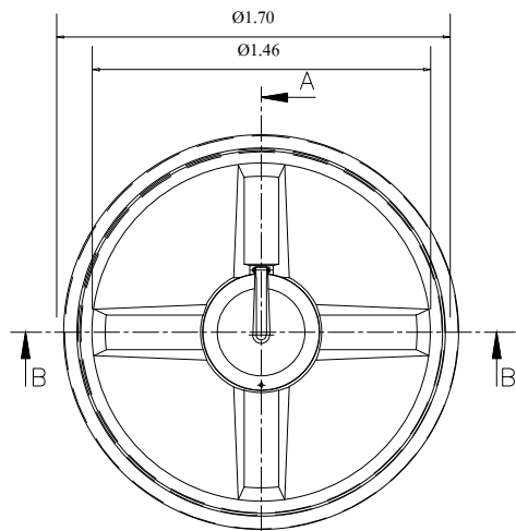
PLAN SCALE 1 : 100
