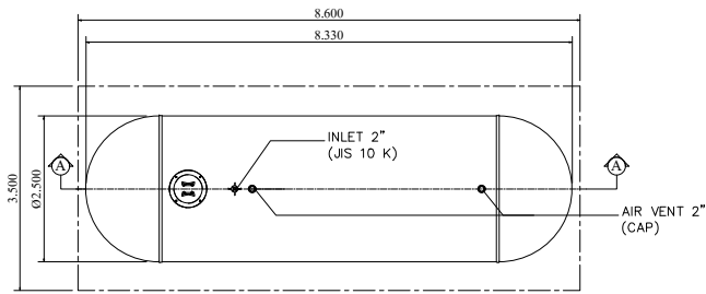
PLAN SCALE : 1:100
