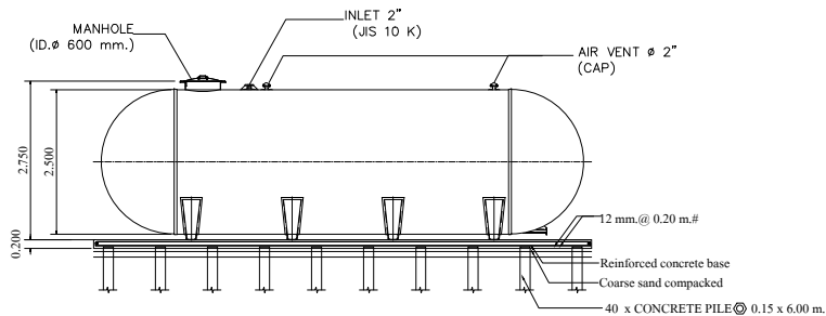
SECTION A - A SCALE : 1:100
