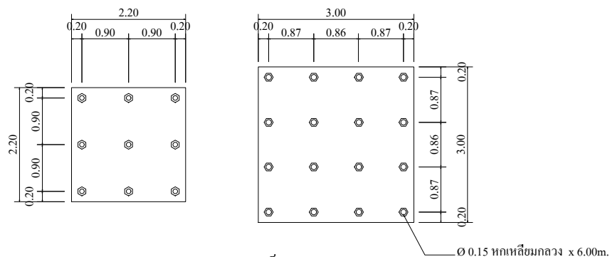
PLAN เส้าเข็ม SCALE 1 : 100
