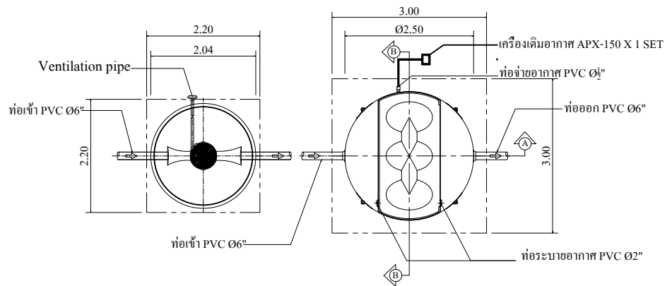
PLAN SCALE 1 : 100
