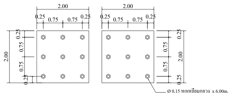
PLAN เสริม SCALE 1 : 100
