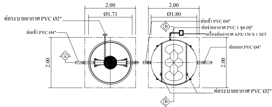
PLAN SCALE 1 : 100
