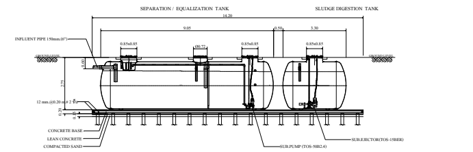
SECTION A-A SCALE 1 : 100
