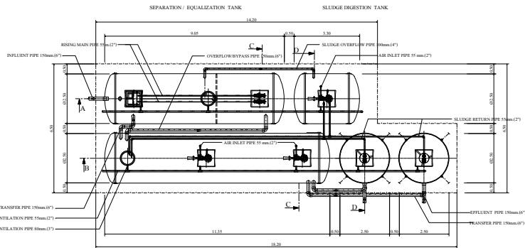
PLAN SCALE 1 : 100
