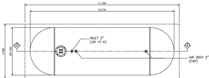
PLAN SCALE : 1:100
