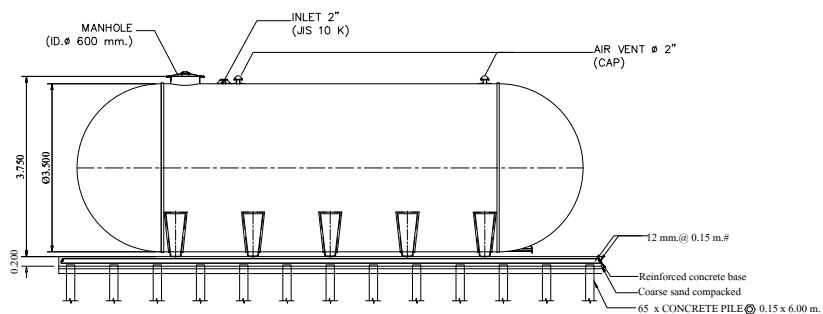
SECTION A - A SCALE : 1:100
