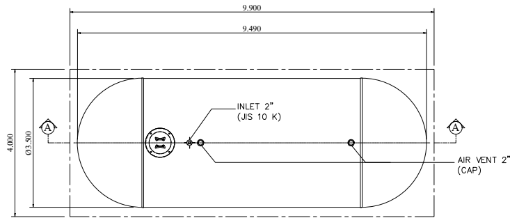
PLAN SCALE : 1:100
