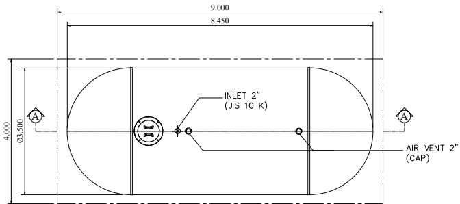
PLAN SCALE : 1:100
