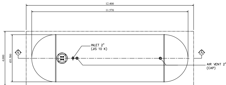
PLAN SCALE : 1:100
