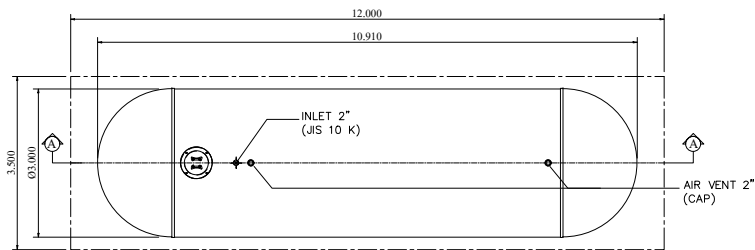
PLAN SCALE : 1:100
