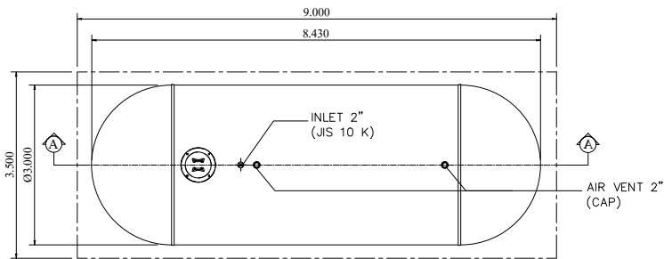
PLAN SCALE : 1:100
