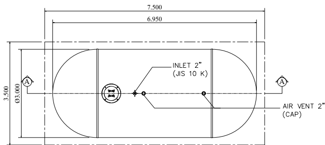
PLAN SCALE : 1:100
