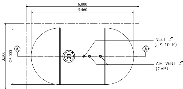
PLAN SCALE : 1:100
