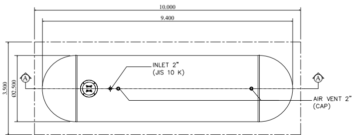
PLAN SCALE : 1:100
