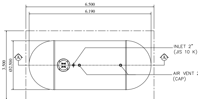
PLAN SCALE : 1:100
