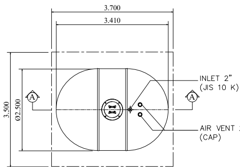
PLAN SCALE : 1:100
