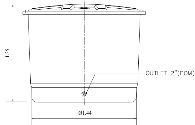
SECTION B-B SCALE 1 : 100
