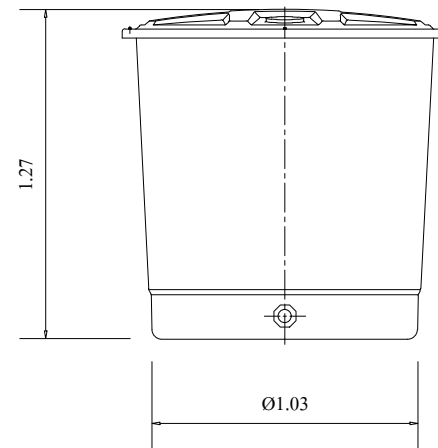
SECTION B-B SCALE 1 : 100
