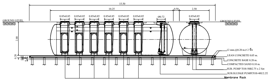
SECTION A-A SCALE 1:100
