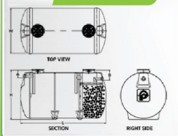
EC-25E to 50E
